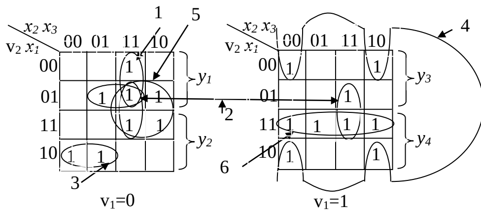
Рис. 3.21. Совместная минимизация функций системы
