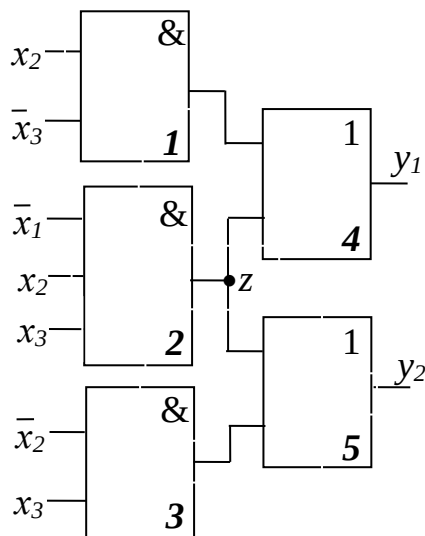
Рис.3.20. Схема, реализующая систему булевых функций.
