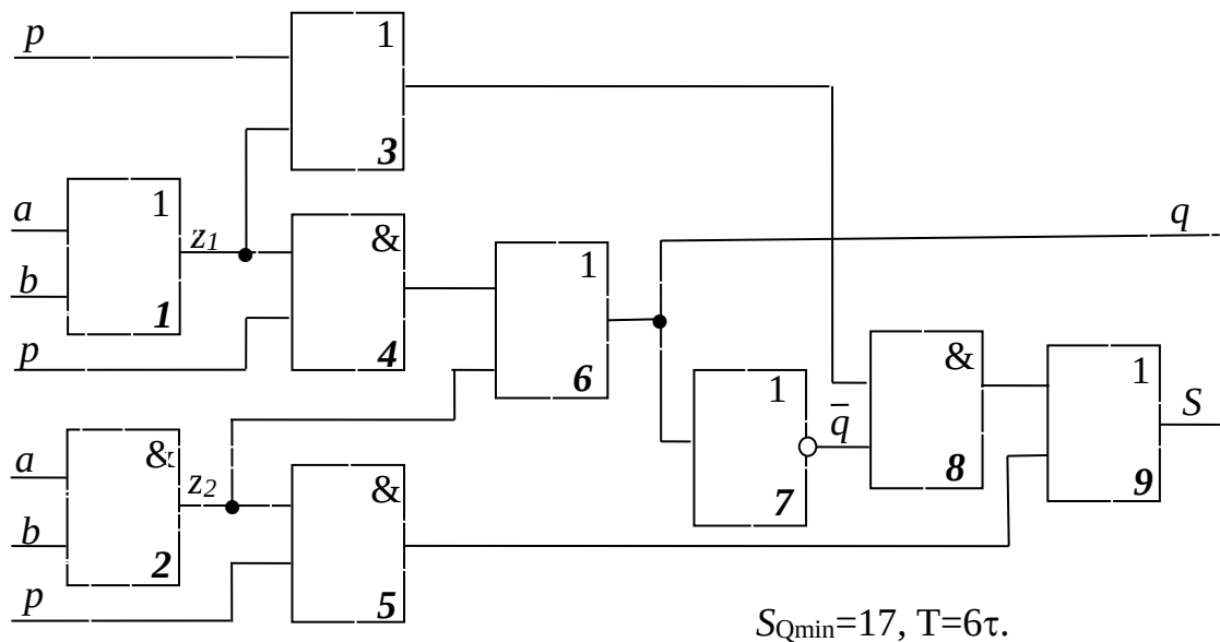
Рис. 3.25. Схема одноразрядного комбинационного сумматора
