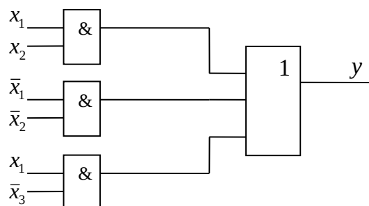
Рис. 2.3. Логическая схема, построенная по покрытию C_2 примера 2.11.
