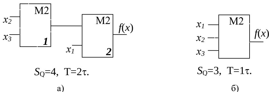
Рис. 3.16. Схемы в базисах Жегалкина: а) на двухвходовых элементах; б) на трехвходовом элементе
