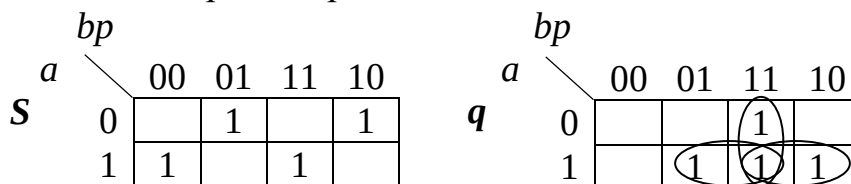
Рис. 3.24. Раздельная минимизация функций системы
