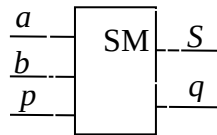
Рис. 3.23. Условно-графическое изображение одноразрядного сумматора
