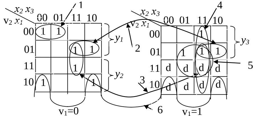
Рис. 3. 22. Минимизация функций системы
