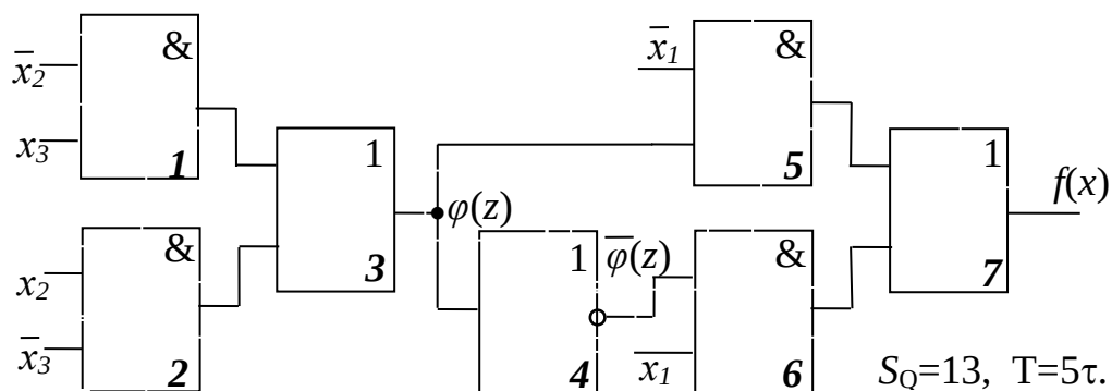
Рис. 3.15. Схема, реализующая систему булевых функций после декомпозиции
