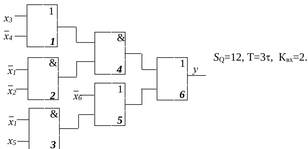
Рис. 3.13. Схема, построенная по выражению (1) с ограничением на число входов в элементы
