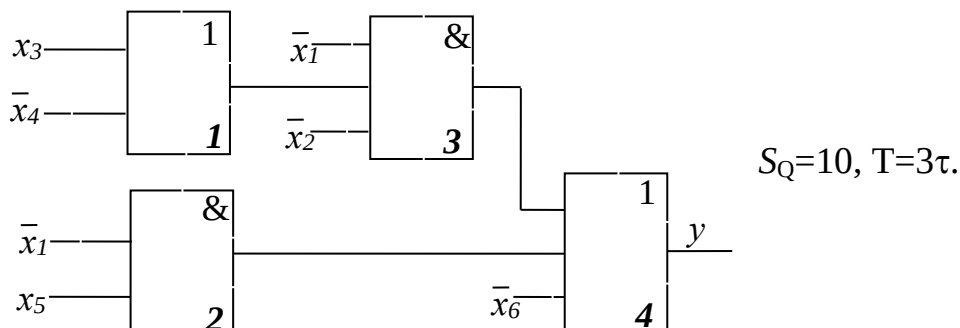
Рис. 3.12. Схема, построенная по выражению после факторного преобразования
